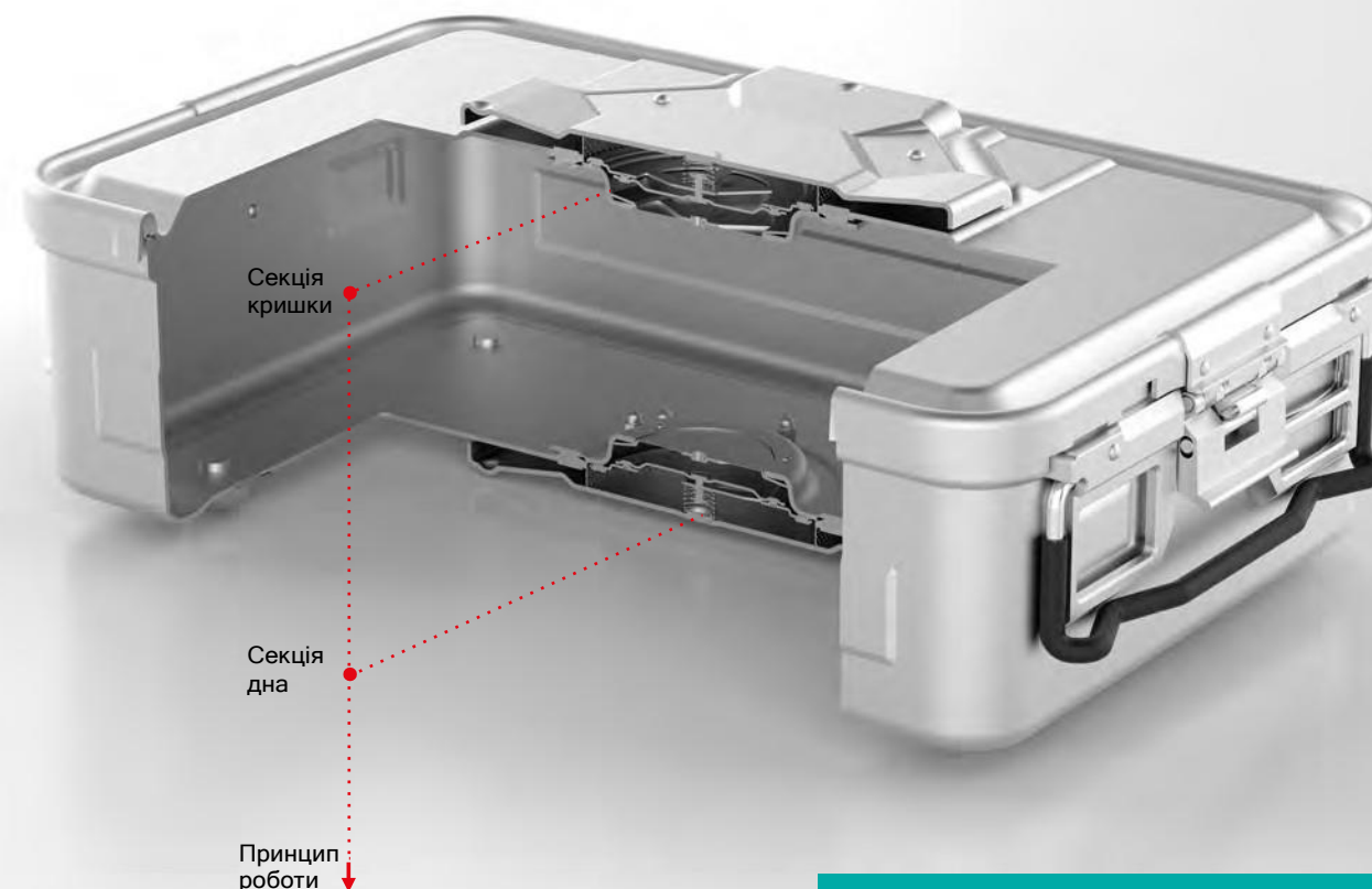
Поперечний розріз механізму та принципи роботи
